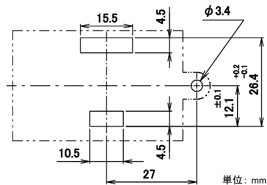
DK1 タブ端子型 (直付タイプ)
