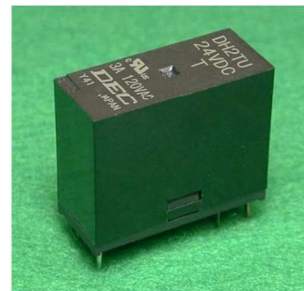
DH2TU (2極クロスパーツイン接点)
