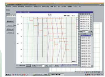
山留め壁の変形 (8図経時変化)
