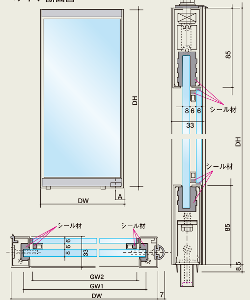
ペアドア断面図
