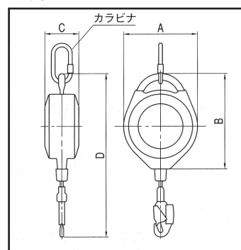
●寸法表 (mm)
