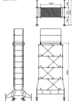
【最高時】
