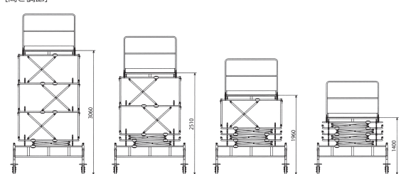
【高さ調節】
