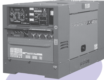
エンジンウェルダー 400A2人用
