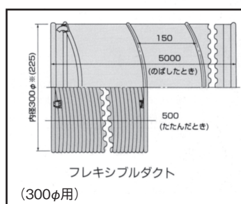
ダクト
